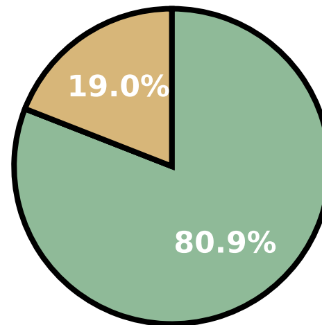
qwen3-max (21)
