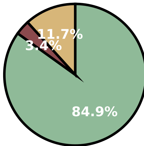
qwen3-32b (179)
