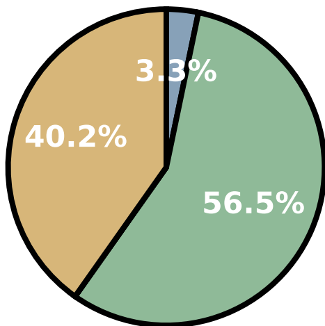
deepseek-v3.2 (92)
