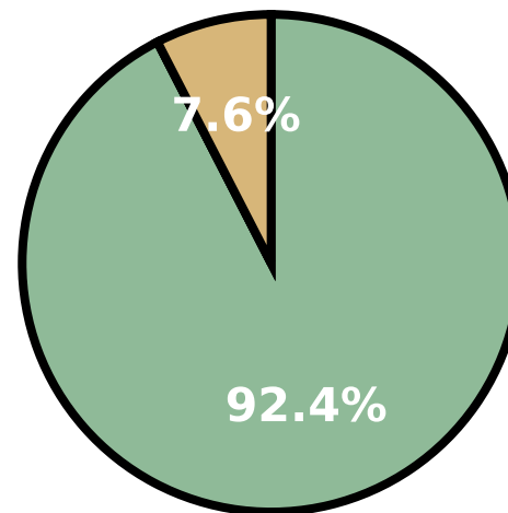
gpt-5.2 (53)
