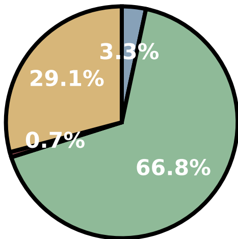
llama3.1:8b (837)
