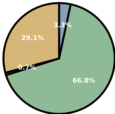
llama3.1:8b
