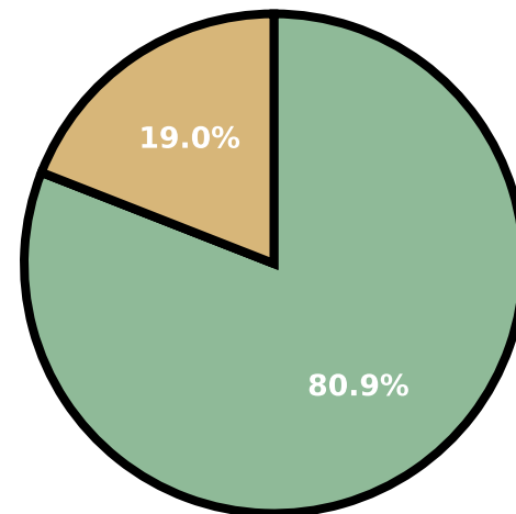
qwen3-max
