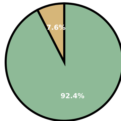
gpt-5.2
