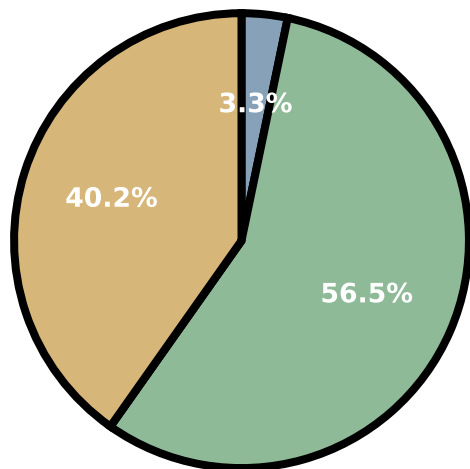
deepseek-v3.2
