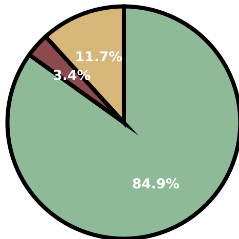
qwen3-32b
