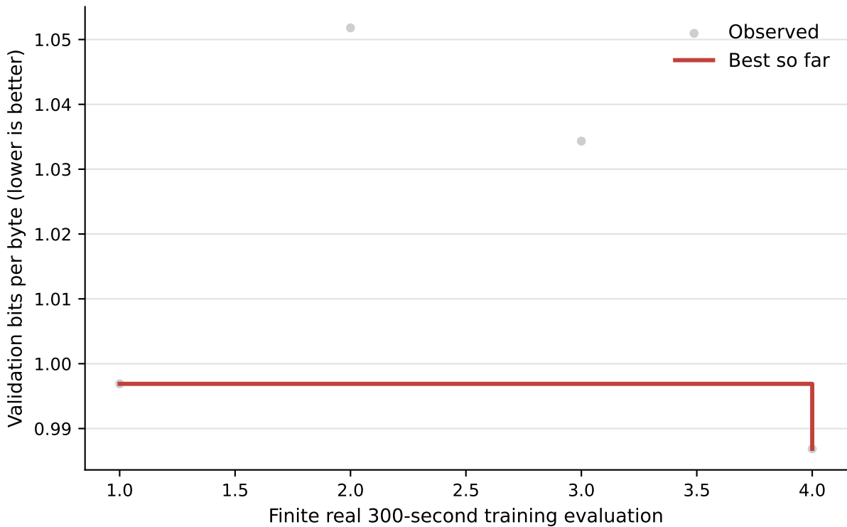
NanoGPT LDM: LCB N4H4 (0/100 interim)
