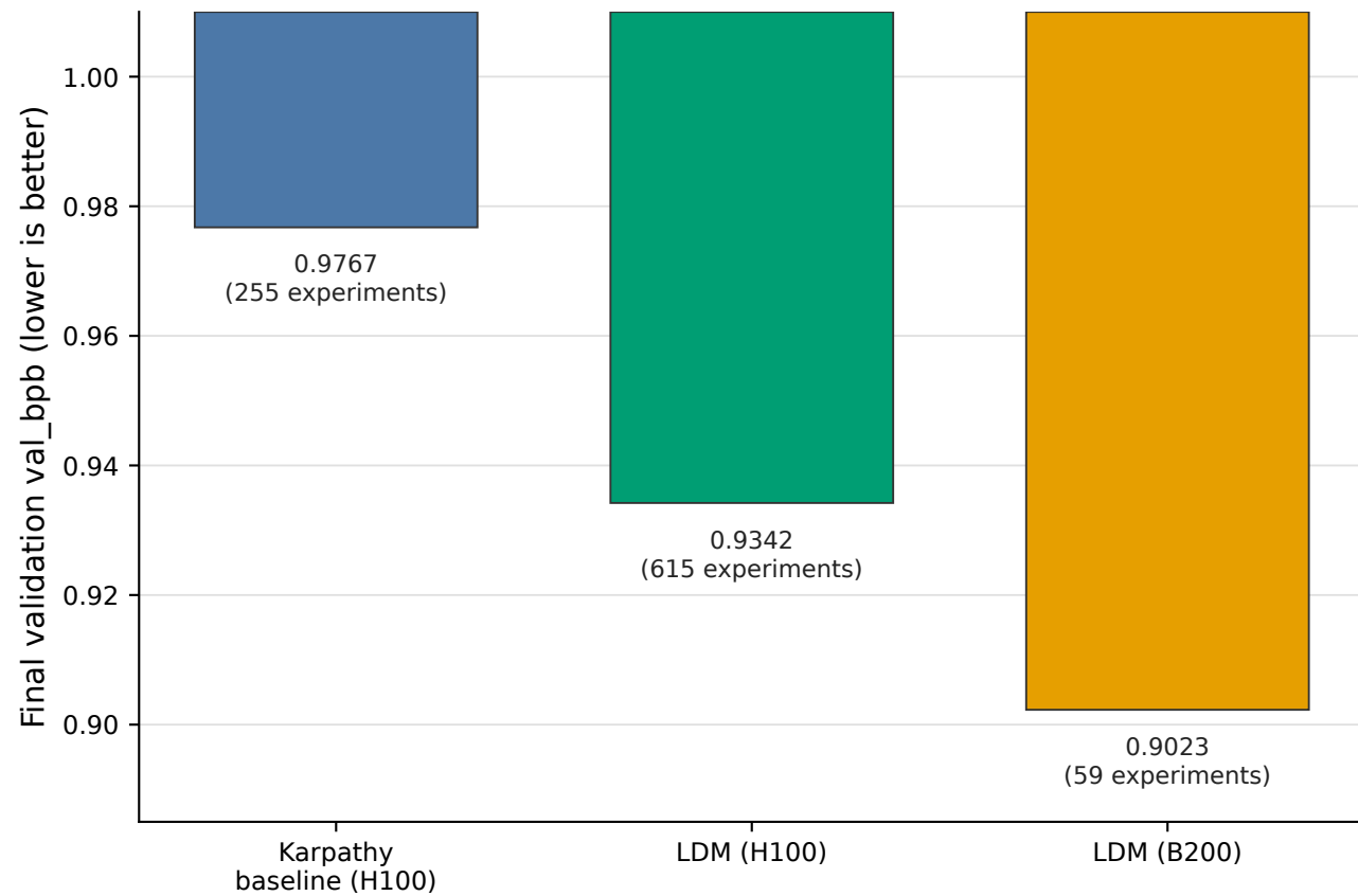
(a) AutoResearch
