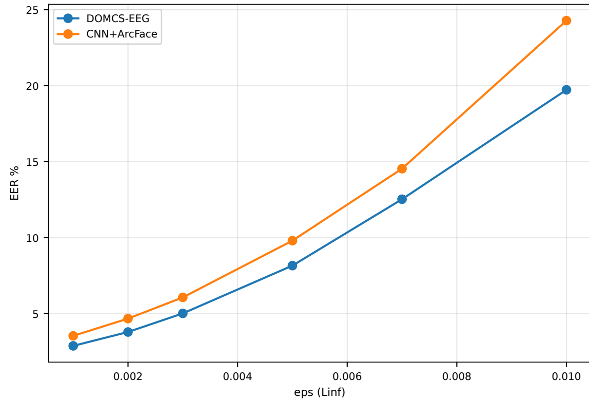
T4 PGD EER vs epsilon
