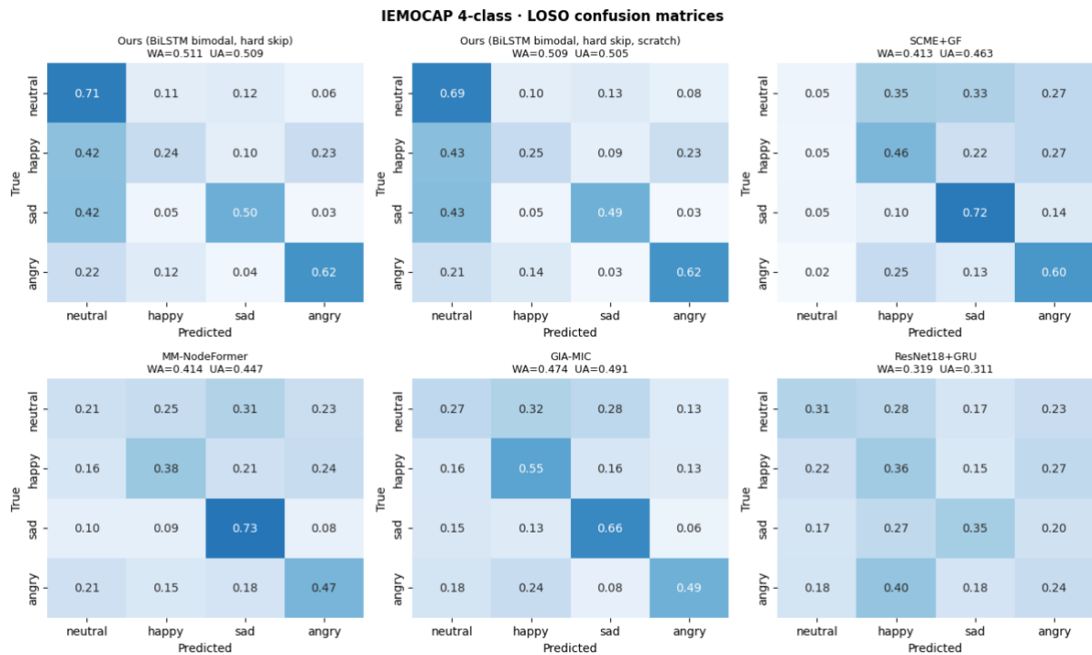
Рисунок 3. Матрица ошибок всех моделей.
