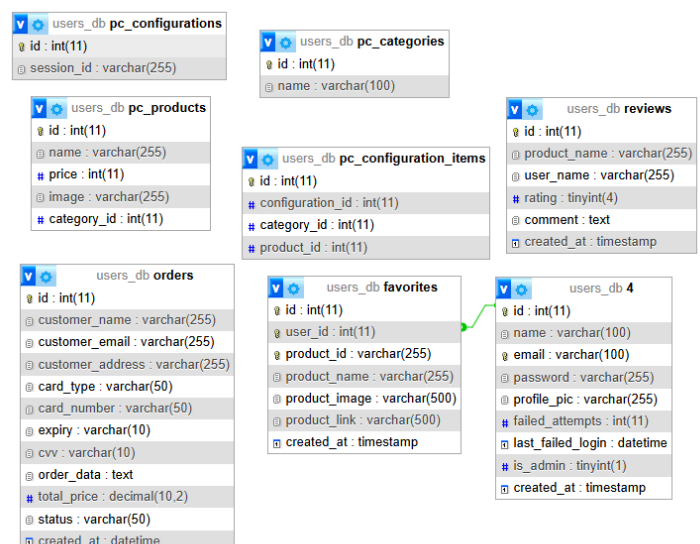
30. ábra: Adatbázis kapcsolatok
