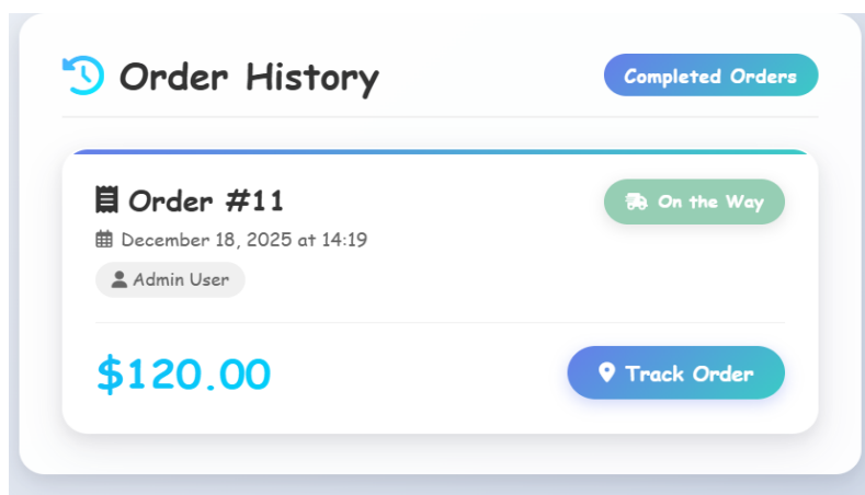
29. ábra: Rendeléseim
