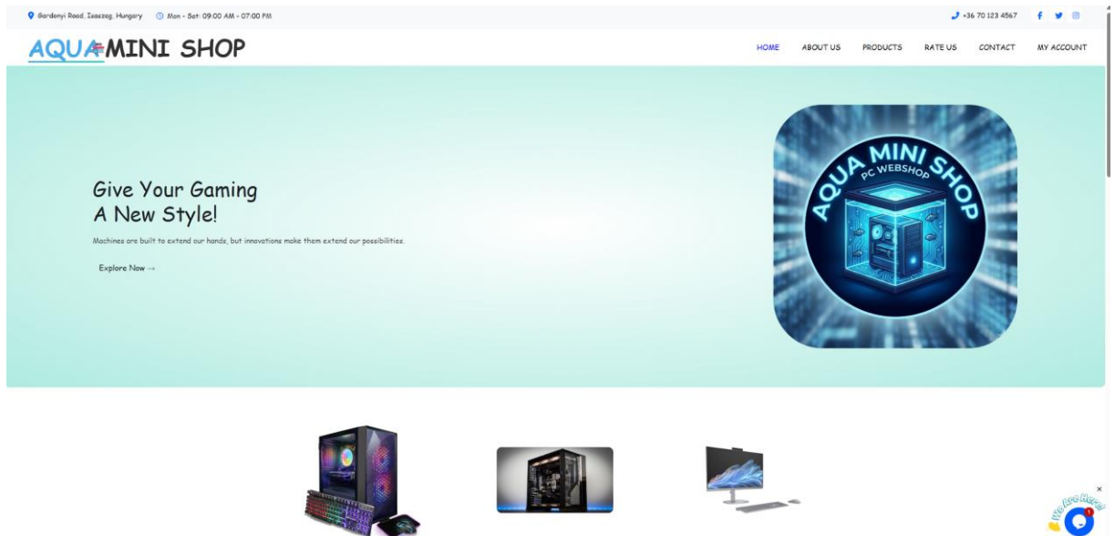
19. ábra: Főoldal
