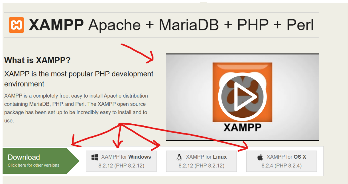
6. ábra: XAMPP
