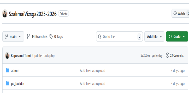
2. ábra: Github
