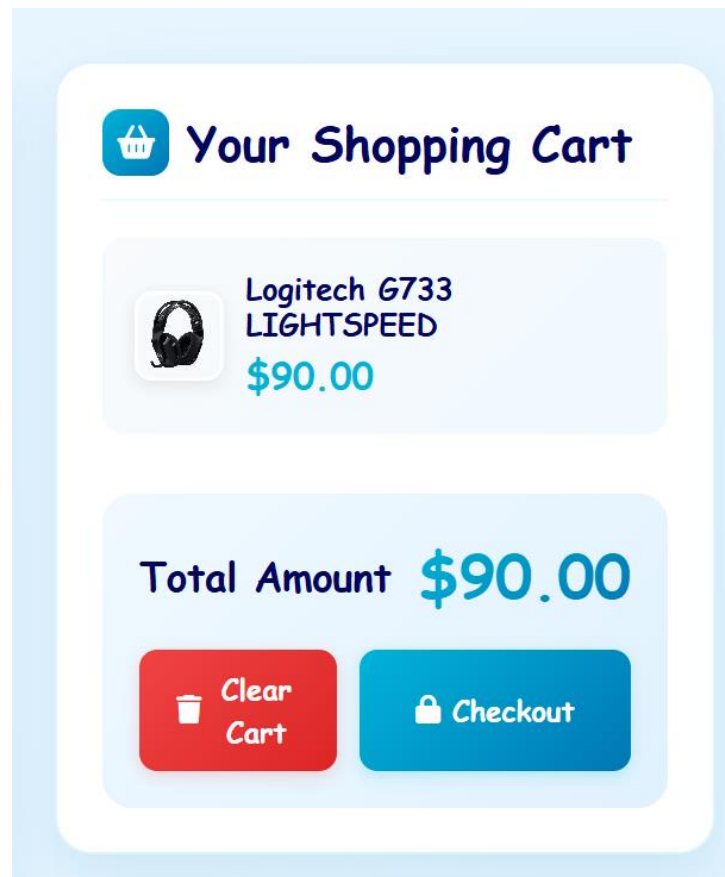
25. ábra: Kosár
