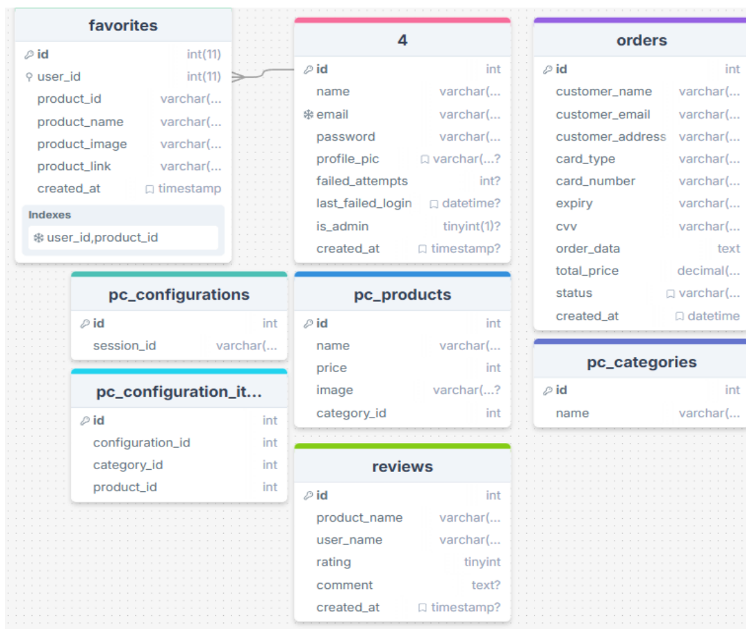
30. ábra: Adatbázis
