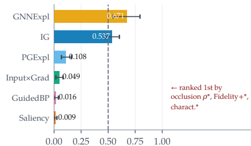
MUTAG-GINE: scaffold shift, n=20
