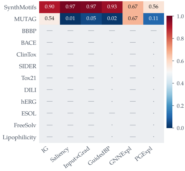
ground-truth localisation (AUROC)
