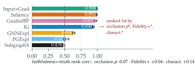
MolMotif-GINE: scaffold shift, n=200
