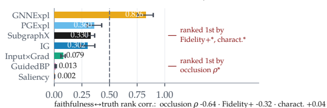
MUTAG-GINE: scaffold shift, n=53
