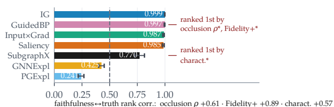
Benzene-GINE: scaffold shift, n=200
