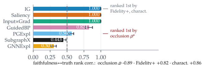
MolMotifHard-GINE: scaffold shift, n=200
