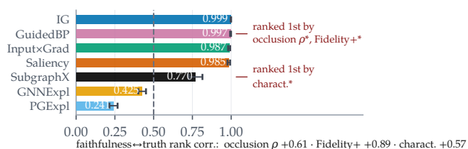
Benzene-GINE: scaffold shift, n=200
