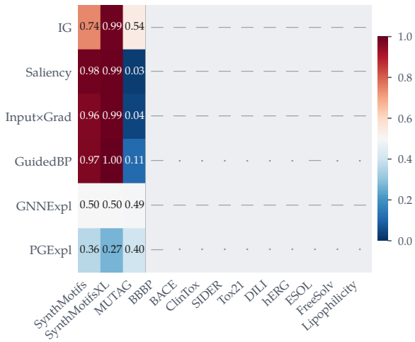
ground-truth localisation (AUROC)
