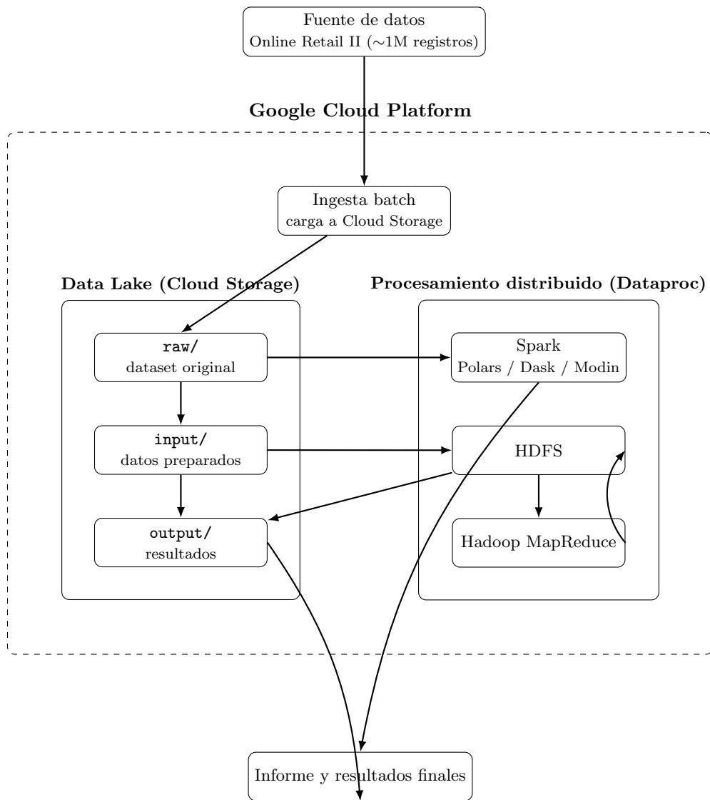
Figura 1: Diagrama de arquitectura general del proyecto
