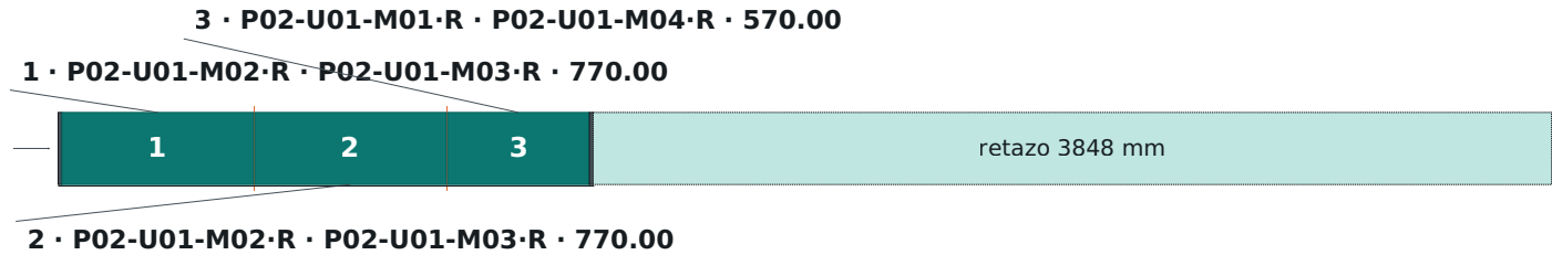
Barra 5 · COMPRA-ACERO-MARCO · 6000.00 mm · retazo reutilizable 3848.00 mm · aprovechamiento 35.2%
