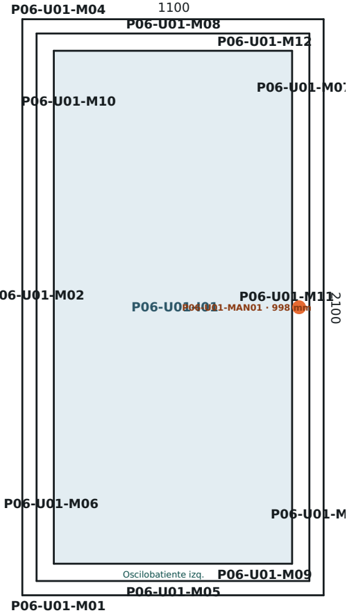
Unidad 1 · Posición P06 · 1 100×2 100 mm · Vista desde interior
