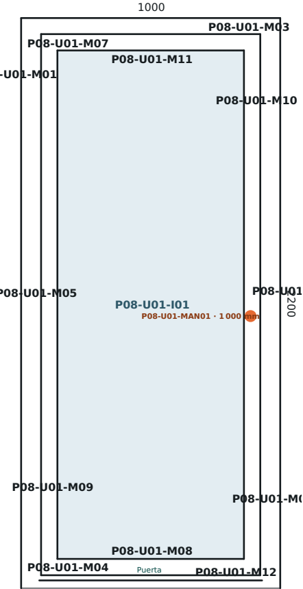
Unidad 1 · Posición P08 · 1000×2 200 mm · Vista desde interior
