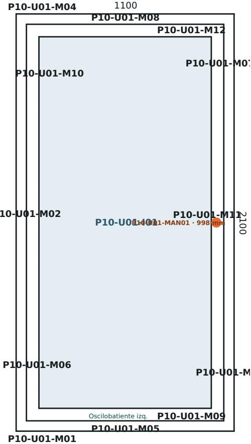
Unidad 1 · Posición P10 · 1 100×2 100 mm · Vista desde interior
