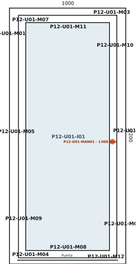
Unidad 1 · Posición P12 · 1000×2 200 mm · Vista desde interior
