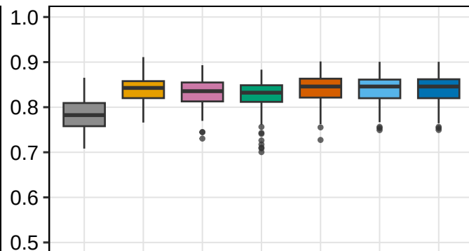
AUC
