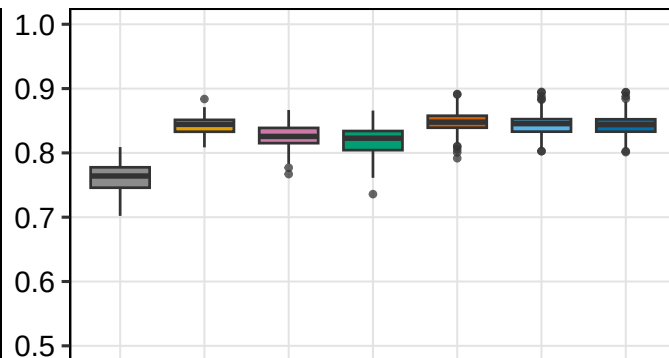
C-index
