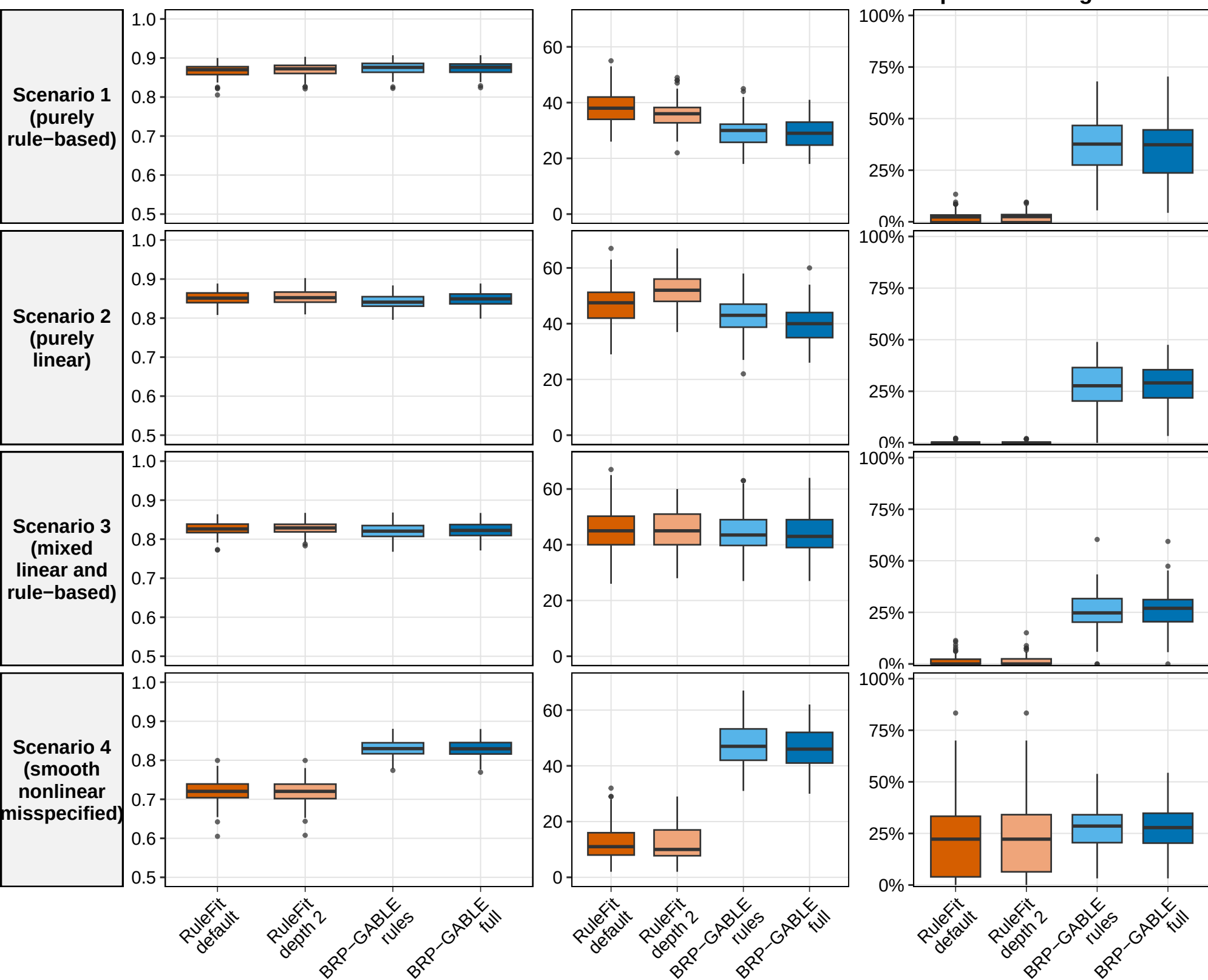
AUC
