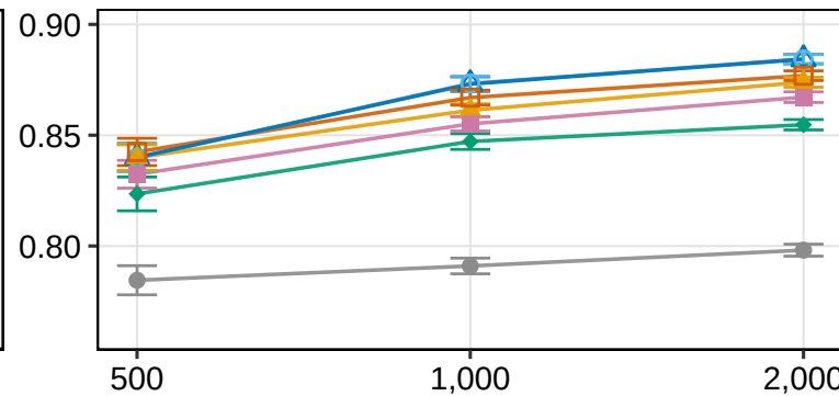
AUC
