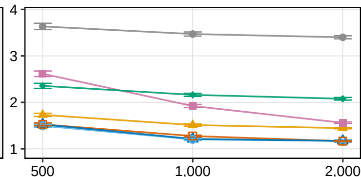
MSE
