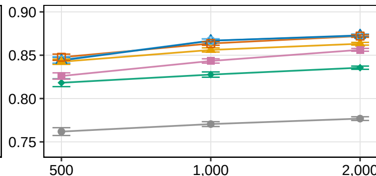
C-index
