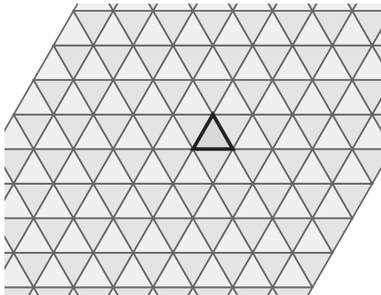
треугольники
