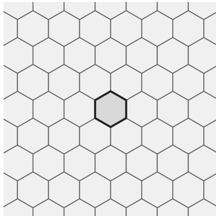
шестиугольники
