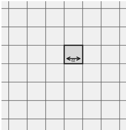
квадраты
