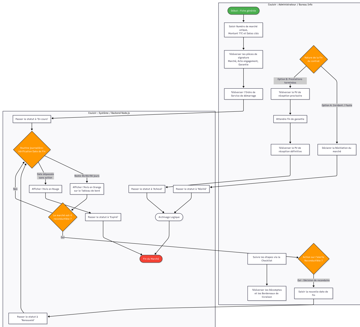
FIGURE 3.5 – Diagramme d’activités : traitement d’un marché
