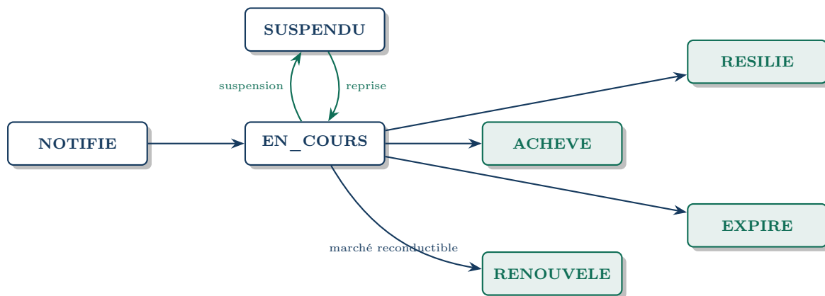
FIGURE 4.5 – Diagramme d'états d'un marché, incluant les transitions de suspension et de reconduction
