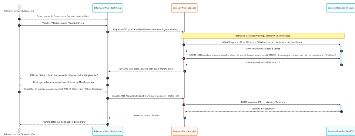
FIGURE 3.7 – Diagramme de séquence : attribution de l'appel d'offres et génération automatique du marché
