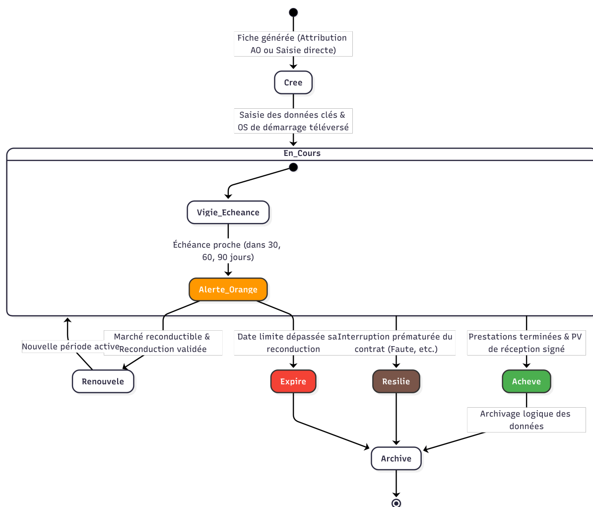
FIGURE 3.9 – Diagramme d'états du marché
