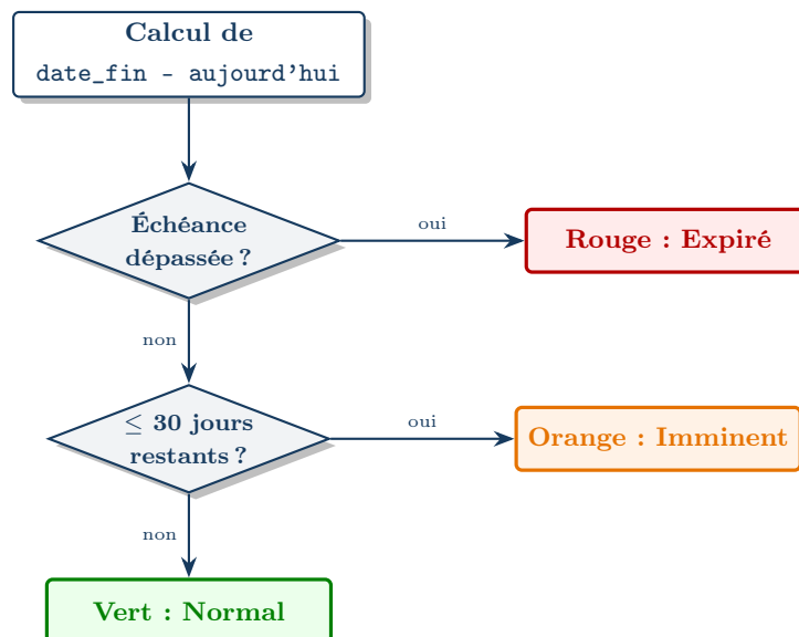
FIGURE 4.9 – Logique de calcul du code couleur des échéances
