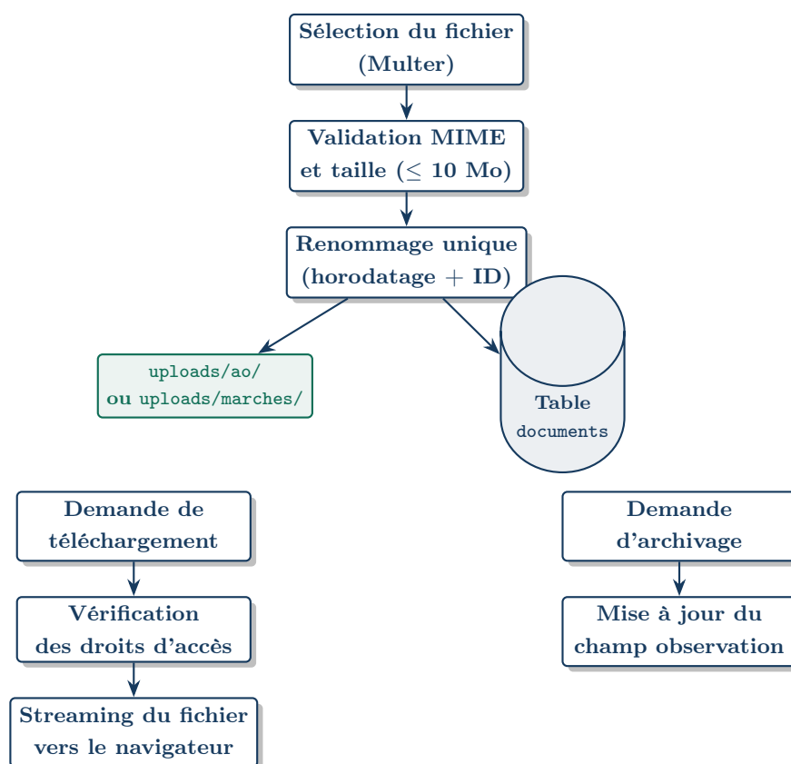
FIGURE 4.6 – Flux de gestion documentaire : téléversement, téléchargement et archivage
