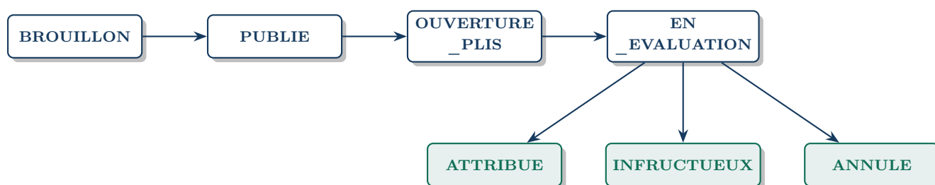
FIGURE 4.4 – Diagramme d'états simplifié d'un appel d'offres
