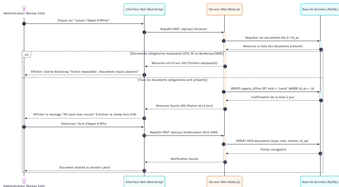
FIGURE 3.6 – Diagramme de séquence : publication d'un appel d'offres avec contrôle documentaire
