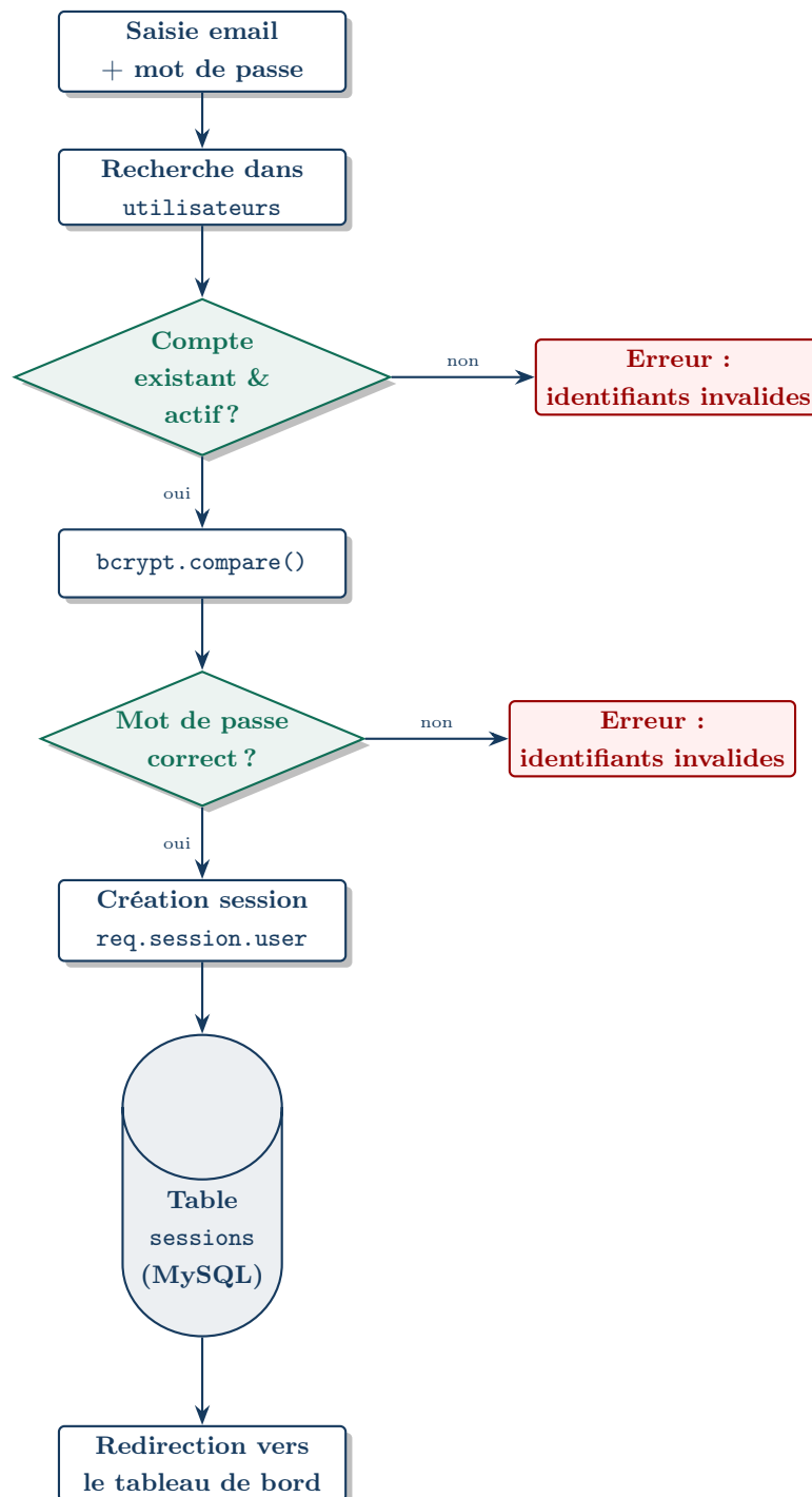
FIGURE 4.1 – Processus d'authentification et de création de session
