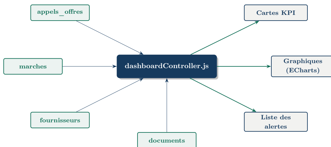
FIGURE 4.2 – Agrégation des données pour l’affichage du tableau de bord
