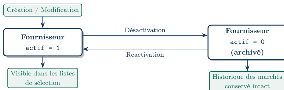
FIGURE 4.3 – Cycle de vie logique d'un fournisseur (suppression douce)
