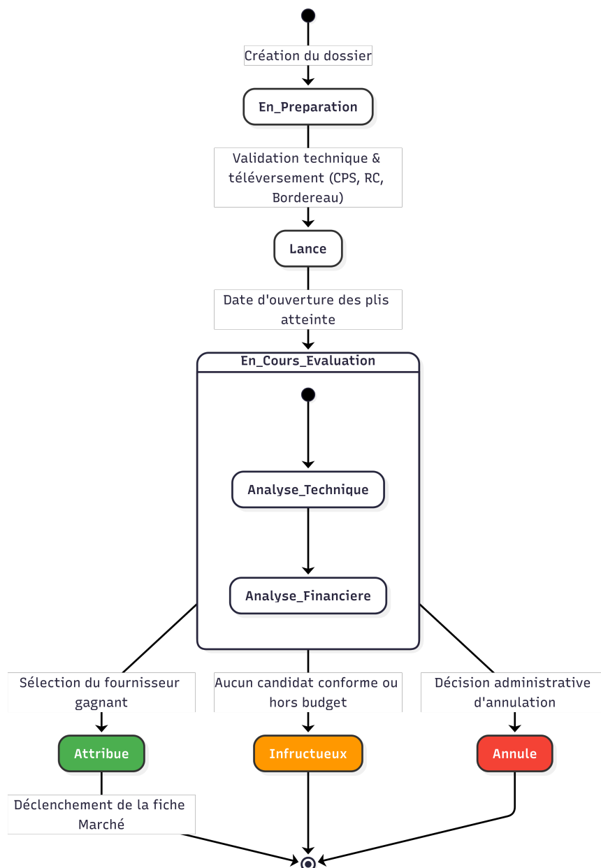
FIGURE 3.8 – Diagramme d'états de l'appel d'offres
