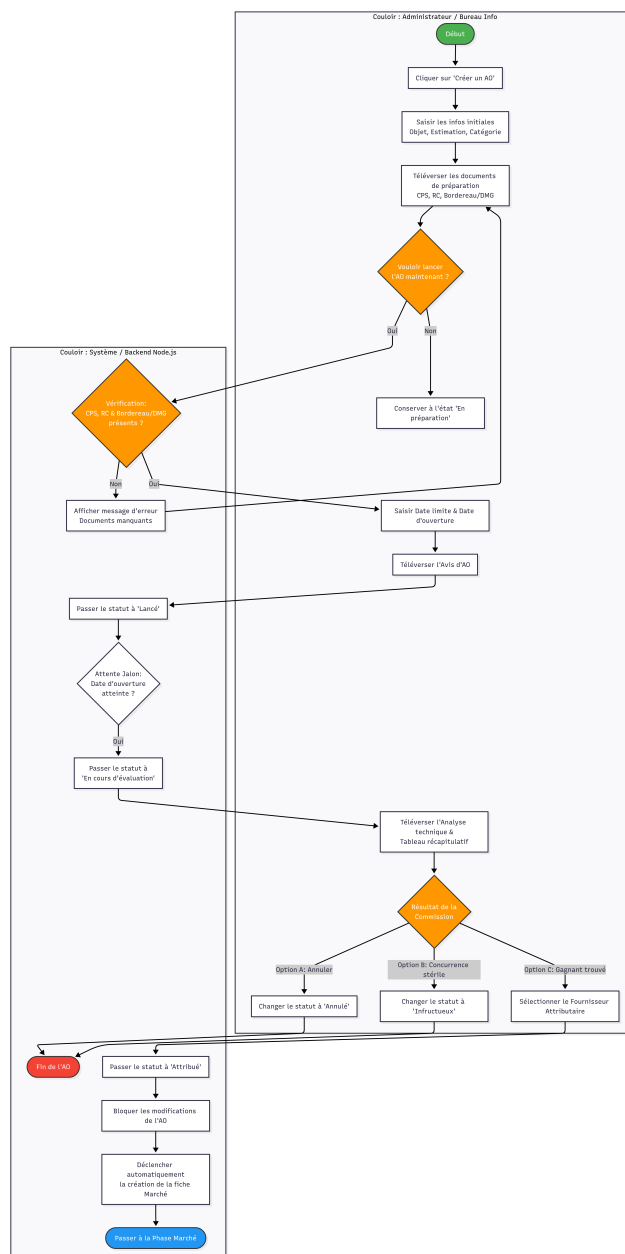
FIGURE 3.4 – Diagramme d'activités : traitement d'un appel d'offres
