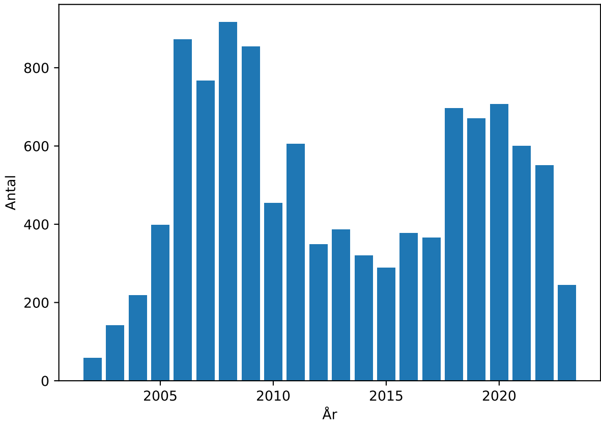
Observations per year — Skogspärlemorfjäril
