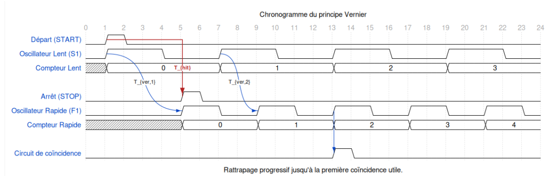
FIGURE 6.1 – Schéma temporel de synthèse du principe Vernier détaillé. Le rattrapage progressif du chemin rapide structure la mesure grossière, tandis que l'observation multiphase affine la position de la première coïncidence dans l'intervalle T_{LSB} .
