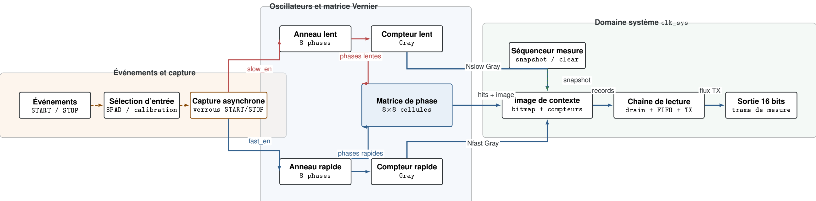
Vue fonctionnelle : les événements arment les anneaux, la matrice fige l'image de mesure, puis la chaîne système lit et émet une trame compacte sur 16 bit.
