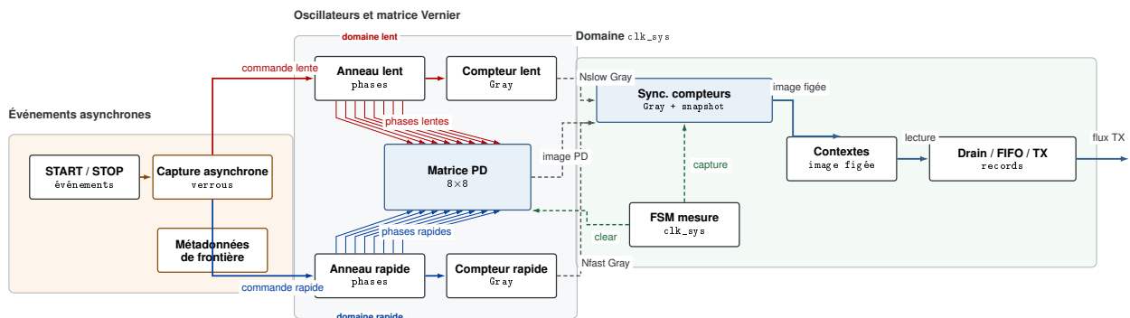
FIGURE 7.2 – Carte des domaines temporels et des traversées CDC de l'architecture MPTDC active.
