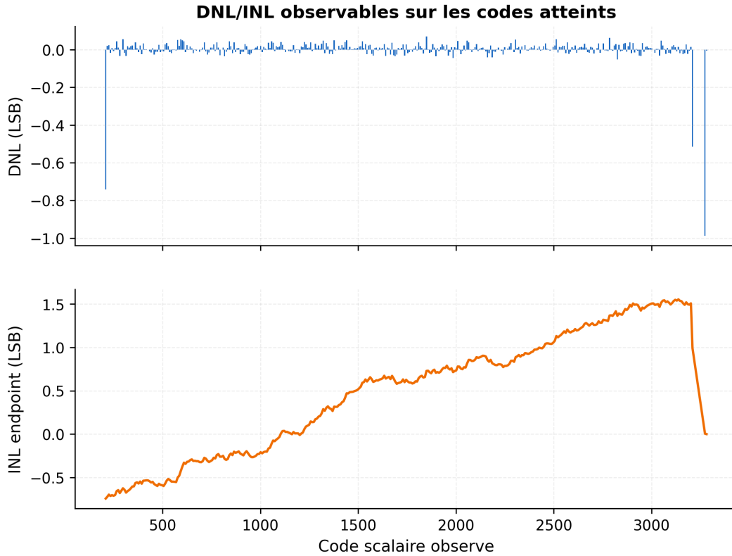
FIGURE 9.2 – DNL et INL observables sur les codes effectivement atteints pendant la campagne.
