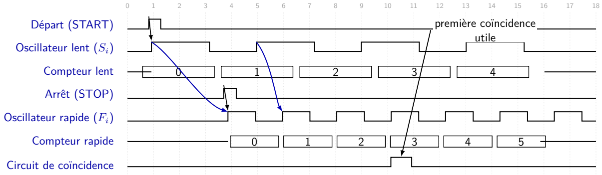
FIGURE 6.1 – Principe Vernier détaillé : rattrapage du chemin rapide, mesure grossière et raffinement multiphase de la coïncidence.
