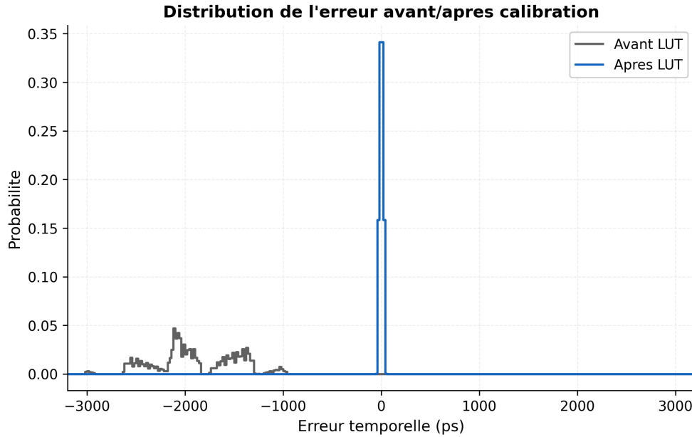
FIGURE 9.1 – Distribution d'erreur avant et après correction LUT externe.
