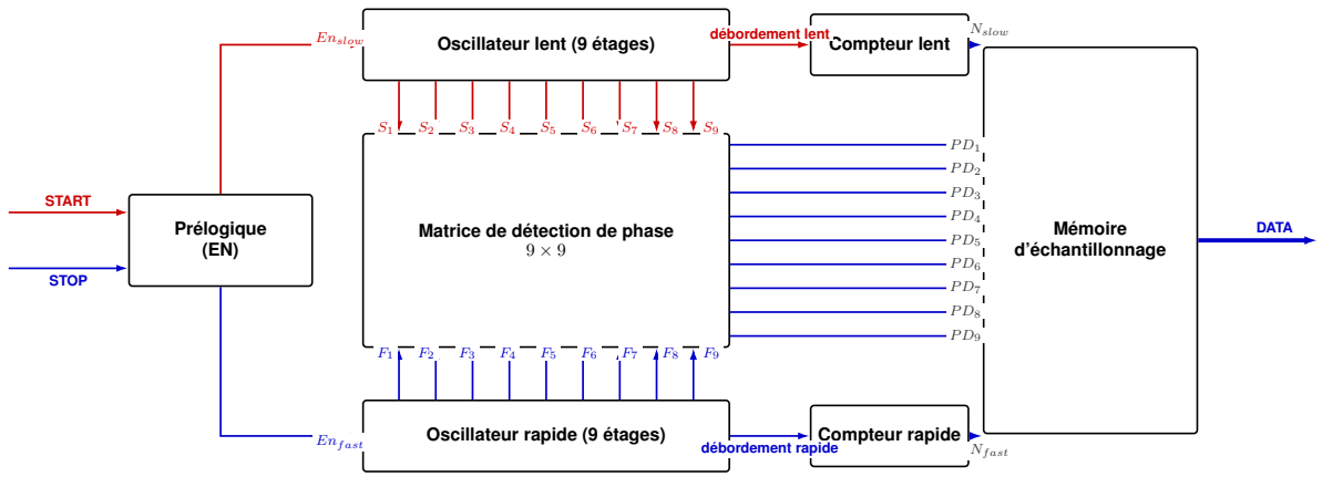
FIGURE 6.2 – Architecture Vernier multiphase de référence, selon les principes décrits dans [2].
