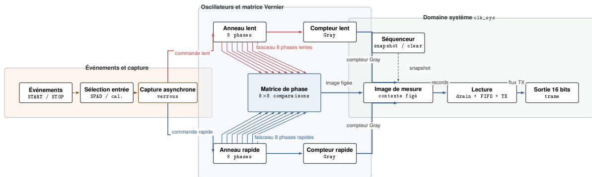
FIGURE 8.2 – Vue fonctionnelle du cœur MPTDC, de la capture START/STOP jusqu'à la lecture compacte en domaine système.
