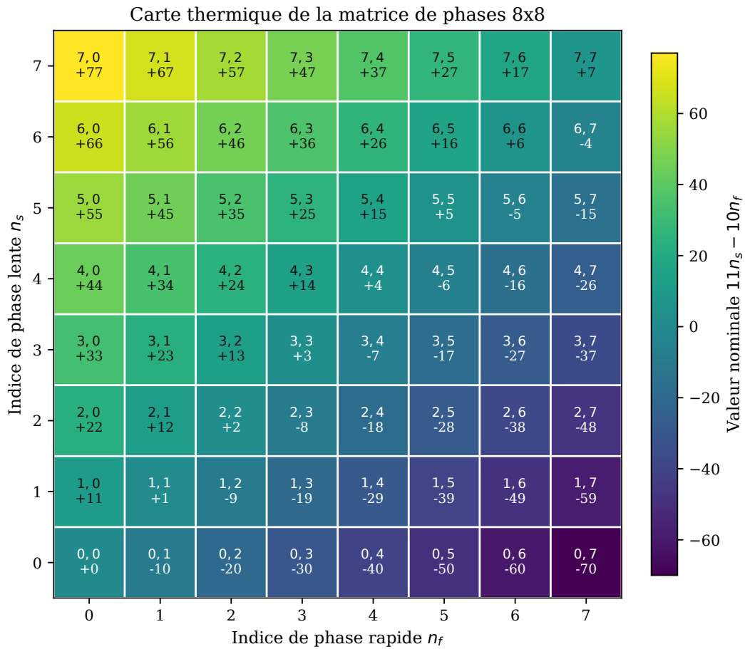
FIGURE 6.4 – Matrice 8 \times 8 des détecteurs de phase et coefficients fins nominaux associés.
