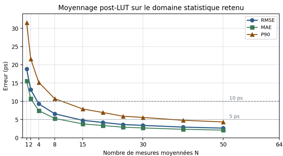
FIGURE 9.3 – Évolution de l'erreur après LUT en fonction du nombre de mesures moyennées.
