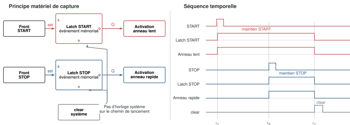
FIGURE 7.4 – Capture asynchrone des événements START/STOP et protection de la fenêtre de mesure par clk_sys .
