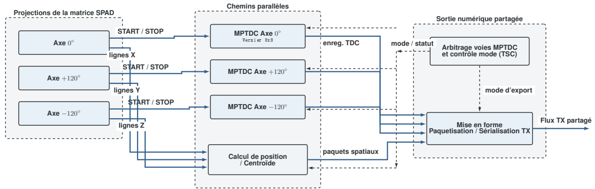
FIGURE 4.1 – Architecture de lecture de SPADMIC et place du chemin temporel MPTDC .
