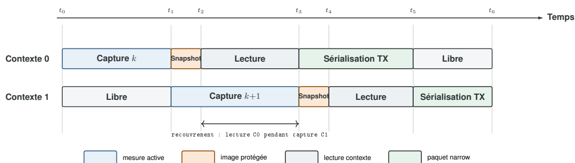
FIGURE 7.5 – Pipeline à deux contextes permettant de recouvrir capture, lecture et sérialisation.
