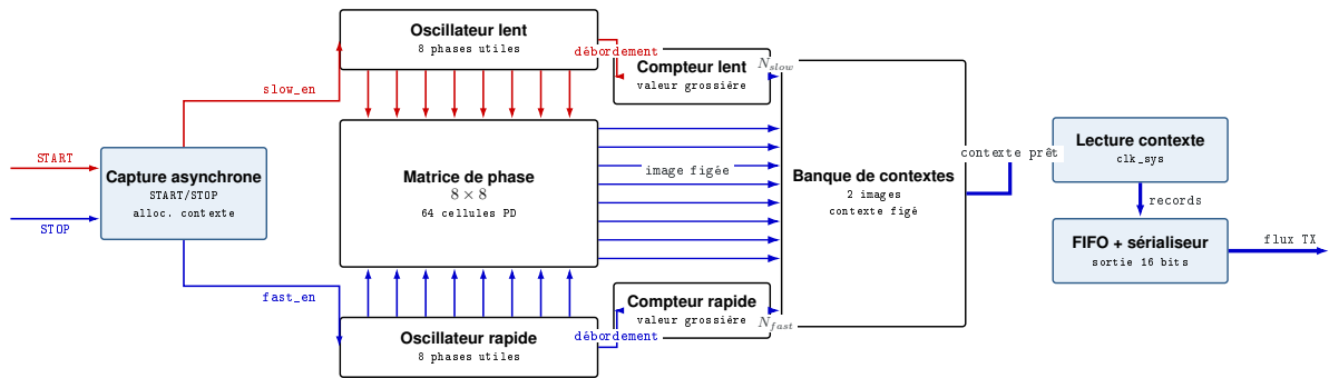
FIGURE 7.1 – Transformation de l'architecture Vernier de référence vers l'implémentation active MPTDC.
