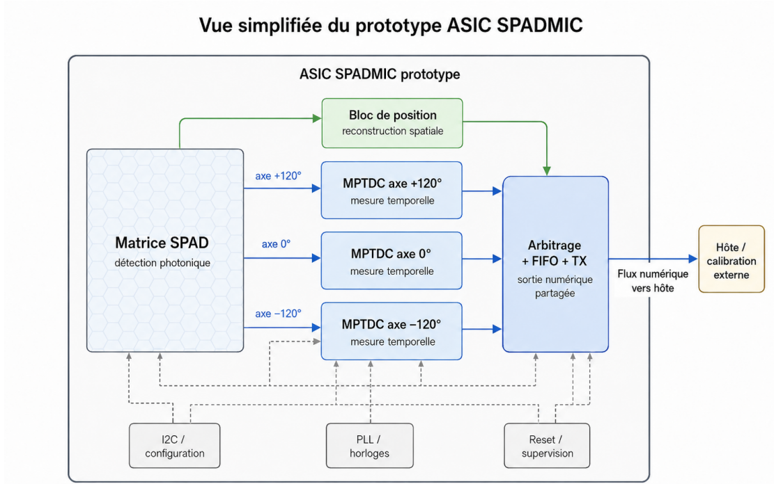
FIGURE 1.1 – Vue d’ensemble du prototype SPADMIC et de la place du cœur MPTDC .
