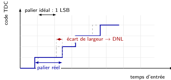
FIGURE 5.2 – Illustration qualitative de la DNL sur une fonction de transfert de TDC.
