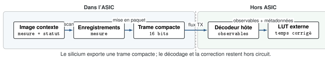
FIGURE 7.6 – Flux de sortie compact et calibration externe par décodage hôte et LUT.
