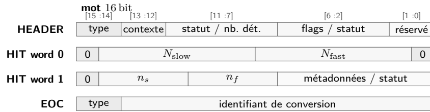
FIGURE 8.5 – Format synthétique de la trame de sortie 16 bit utilisée pour exporter les enregistrements de détection.
