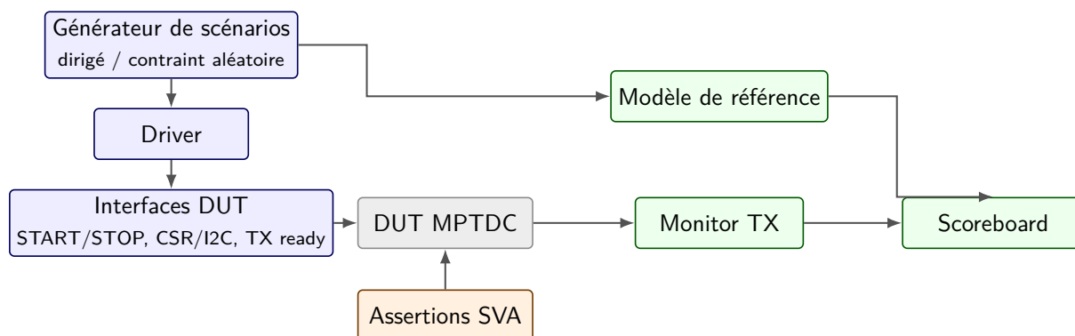
FIGURE 8.6 – Vue simplifiée de l'environnement de vérification fonctionnelle du MPTDC.
