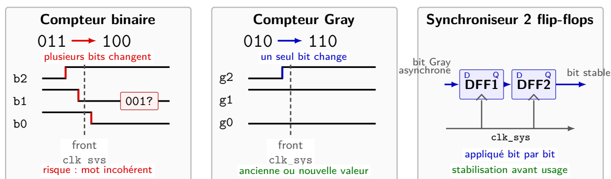
FIGURE 7.3 – Principe de traversée CDC d'un compteur : risque du codage binaire, intérêt du Gray et synchronisation par deux flip-flops.
