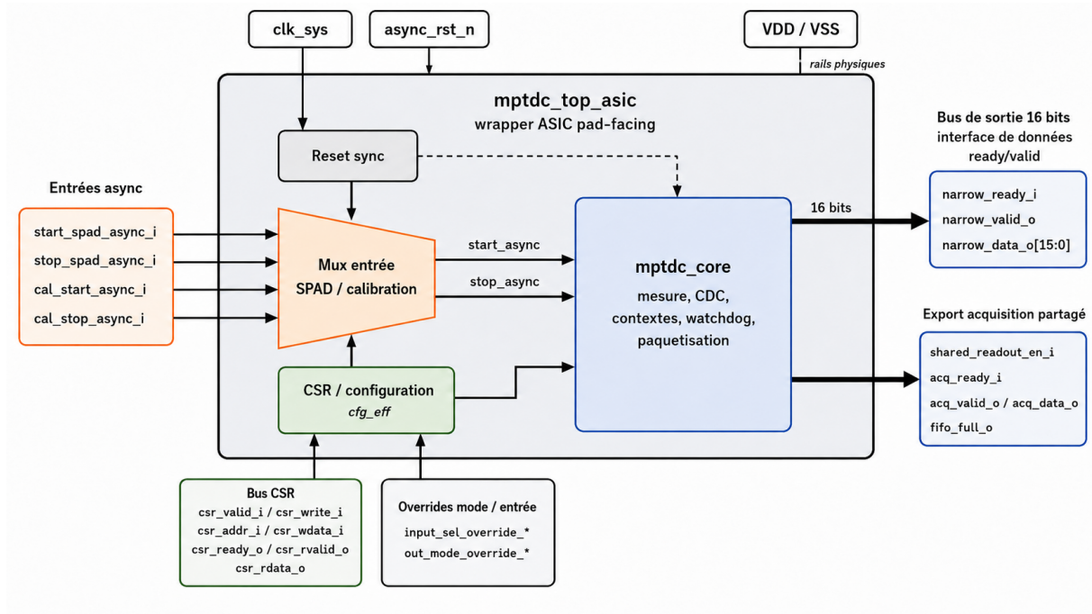
FIGURE 8.1 – Vue top-level du wrapper ASIC MPTDC et de ses interfaces fonctionnelles principales.
