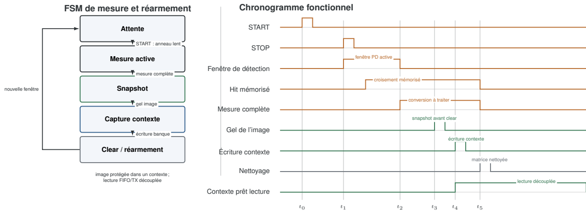
FIGURE 8.3 – Protocole de fermeture d'une mesure, du gel de l'image au nettoyage de la fenêtre de détection.
