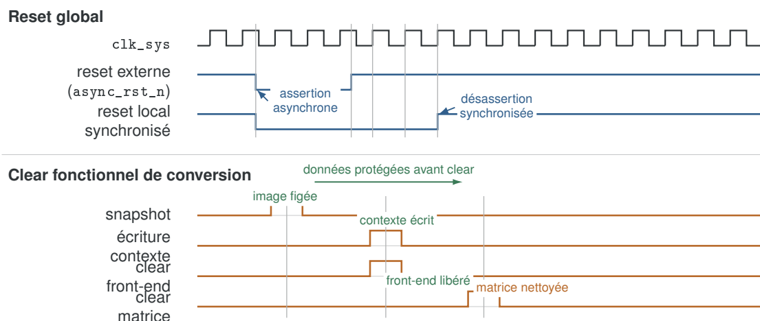
FIGURE 8.4 – Reset global et clear de conversion. Le reset est asserté immédiatement puis relâché de façon synchronisée ; le clear intervient seulement après snapshot et écriture du contexte.
