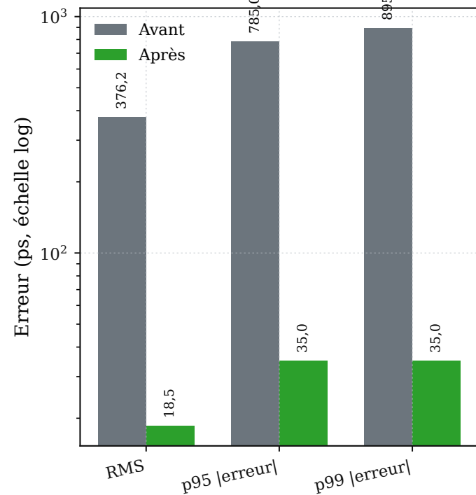
Réduction d'erreur sur validation
