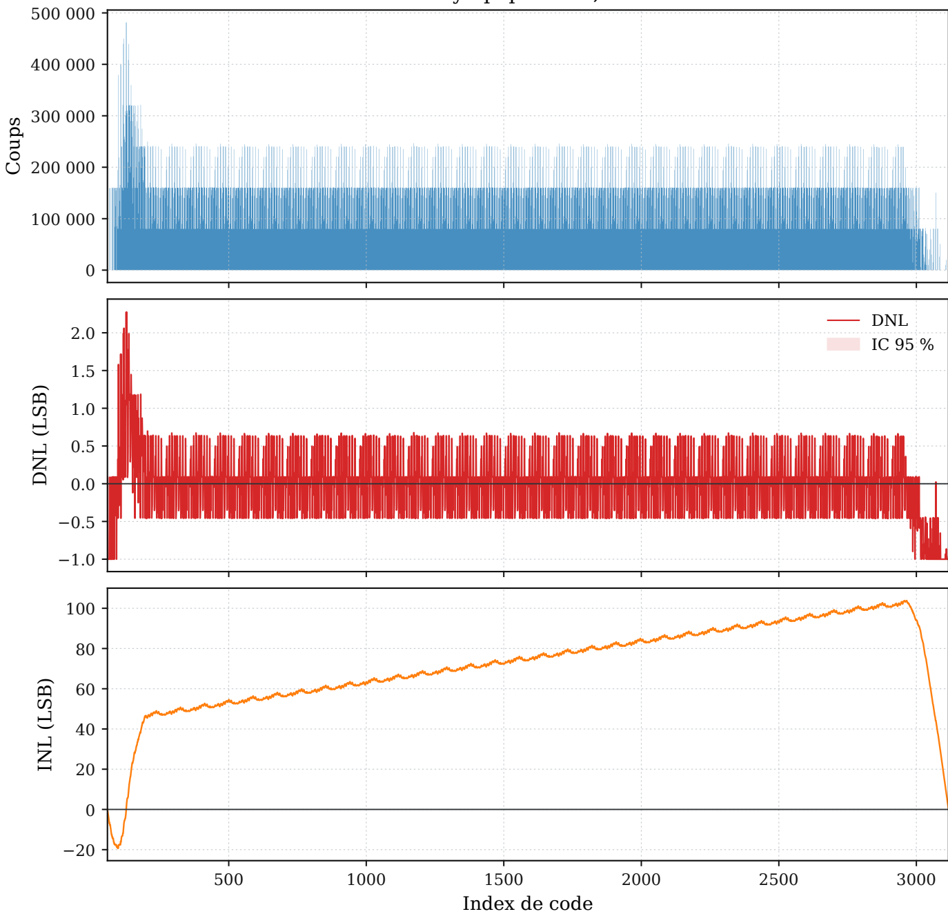
Code-density : population, DNL et INL
