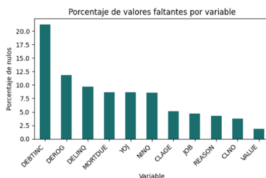
Gráfica 1. Porcentaje de missing values por variable
