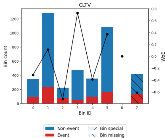
Gráfico 10. Optimal Binning cltv
