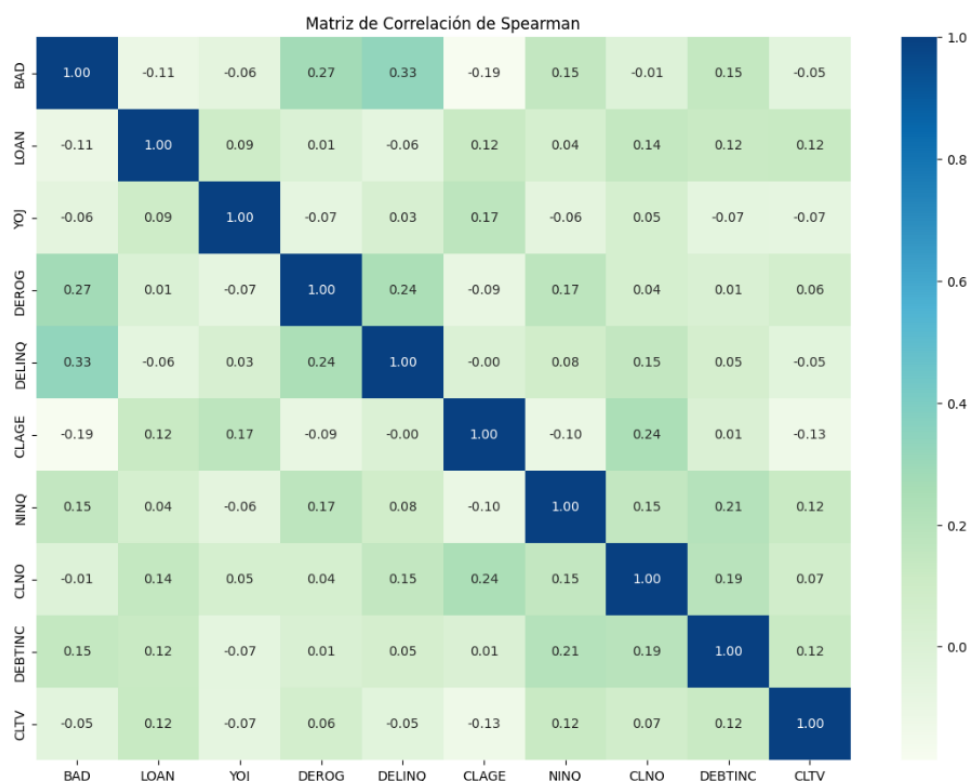
Gráfico 7. Matriz de correlación de Spearman + CLTV
