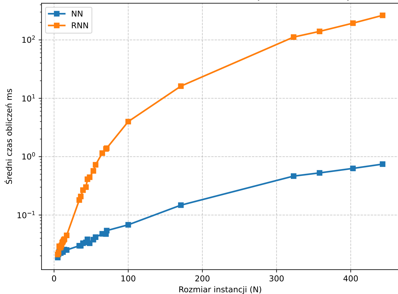
Czas obliczeń dla NN i RNN w funkcji wielkości instancji
