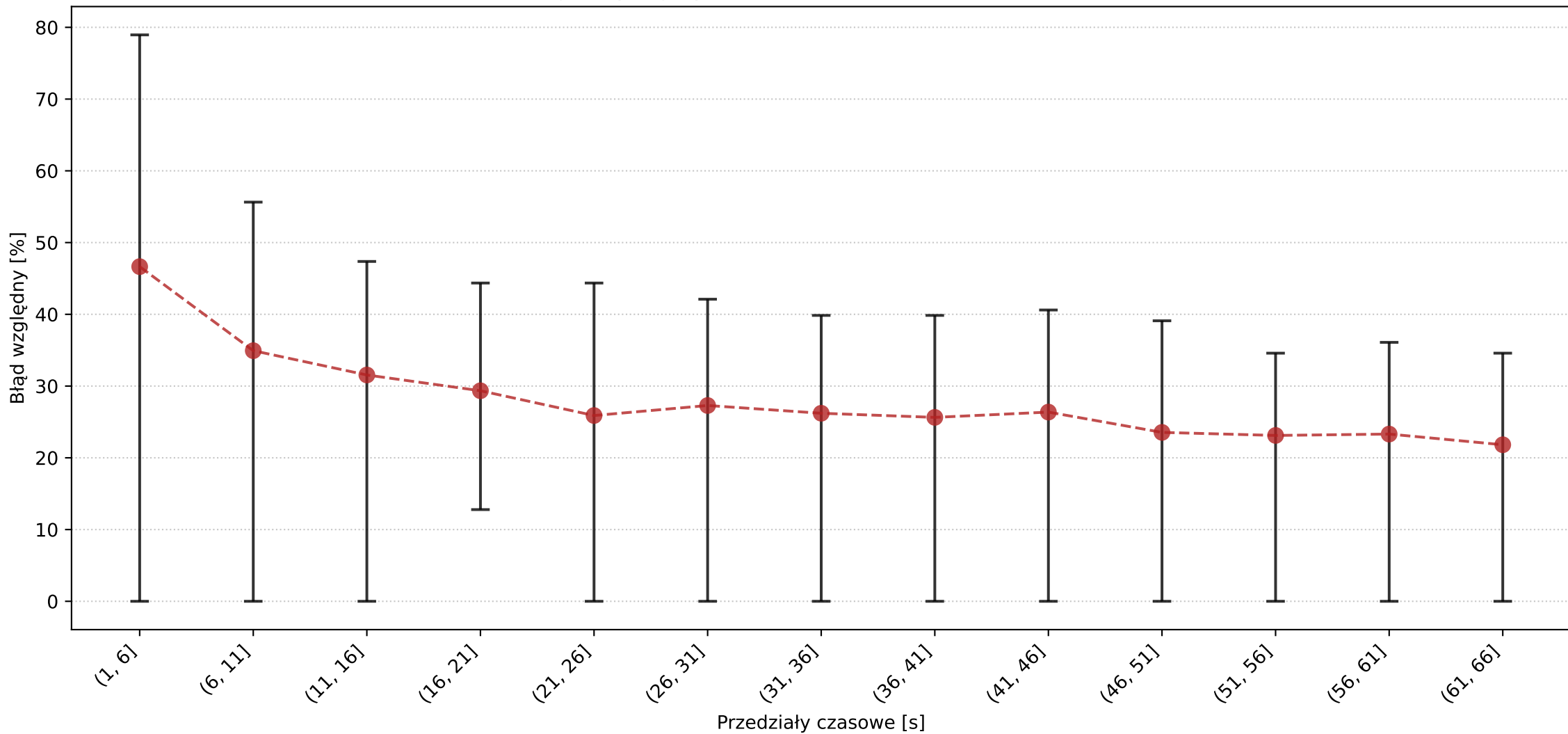
Średni błąd względny algorytmu RAND w czasie z rozrzutem Min-Max (N=14)
