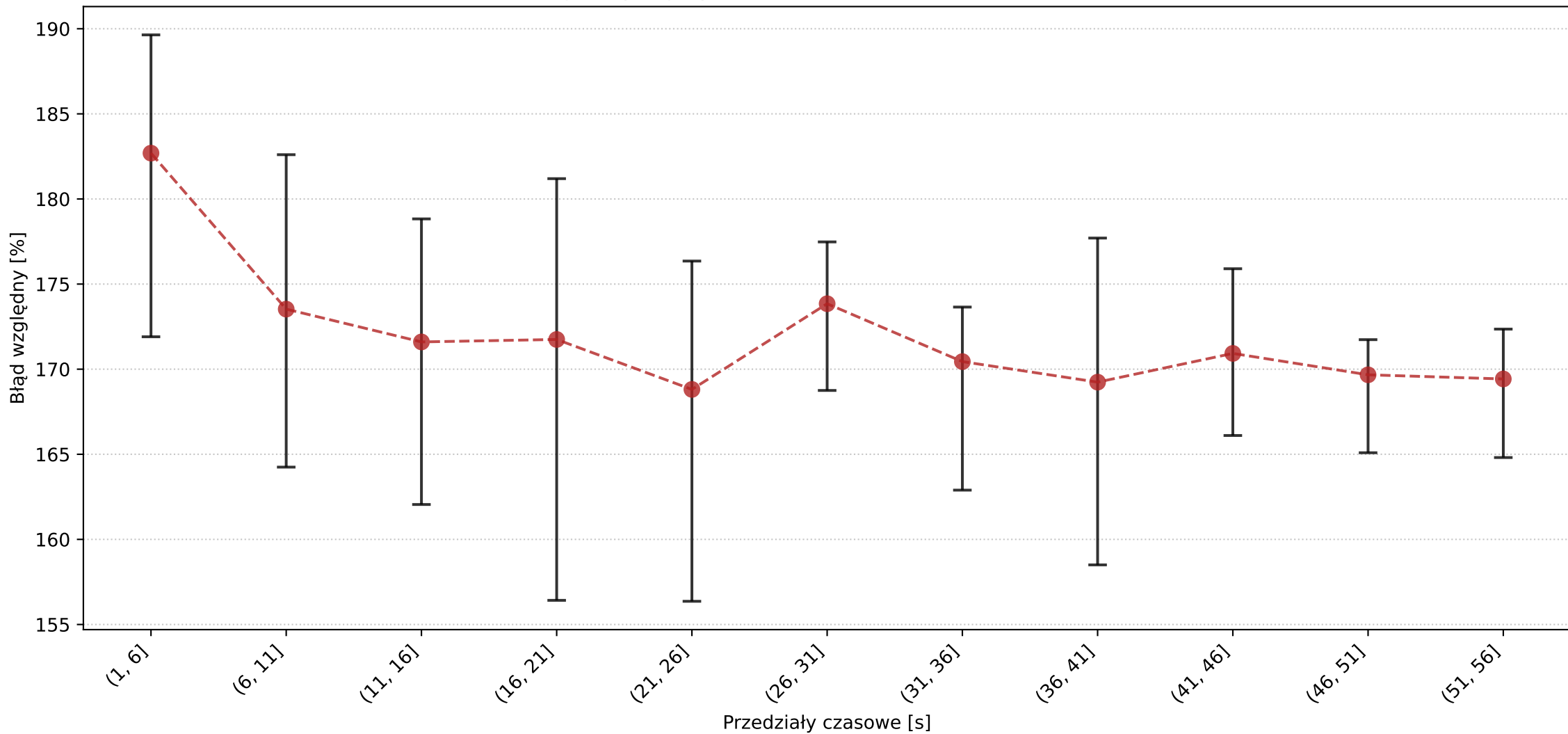
Średni błąd względny algorytmu RAND w czasie z rozrzutem Min-Max (N=48)
