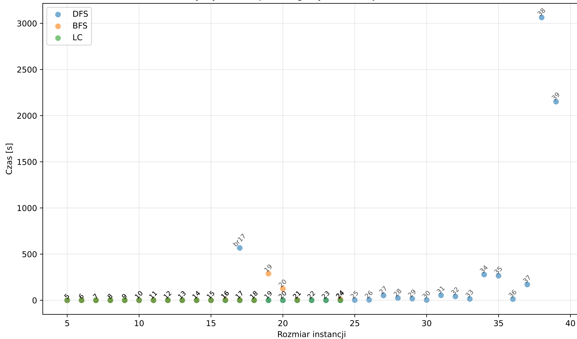
Czasy wykonania poszczególnych instancji (skala liniowa)
