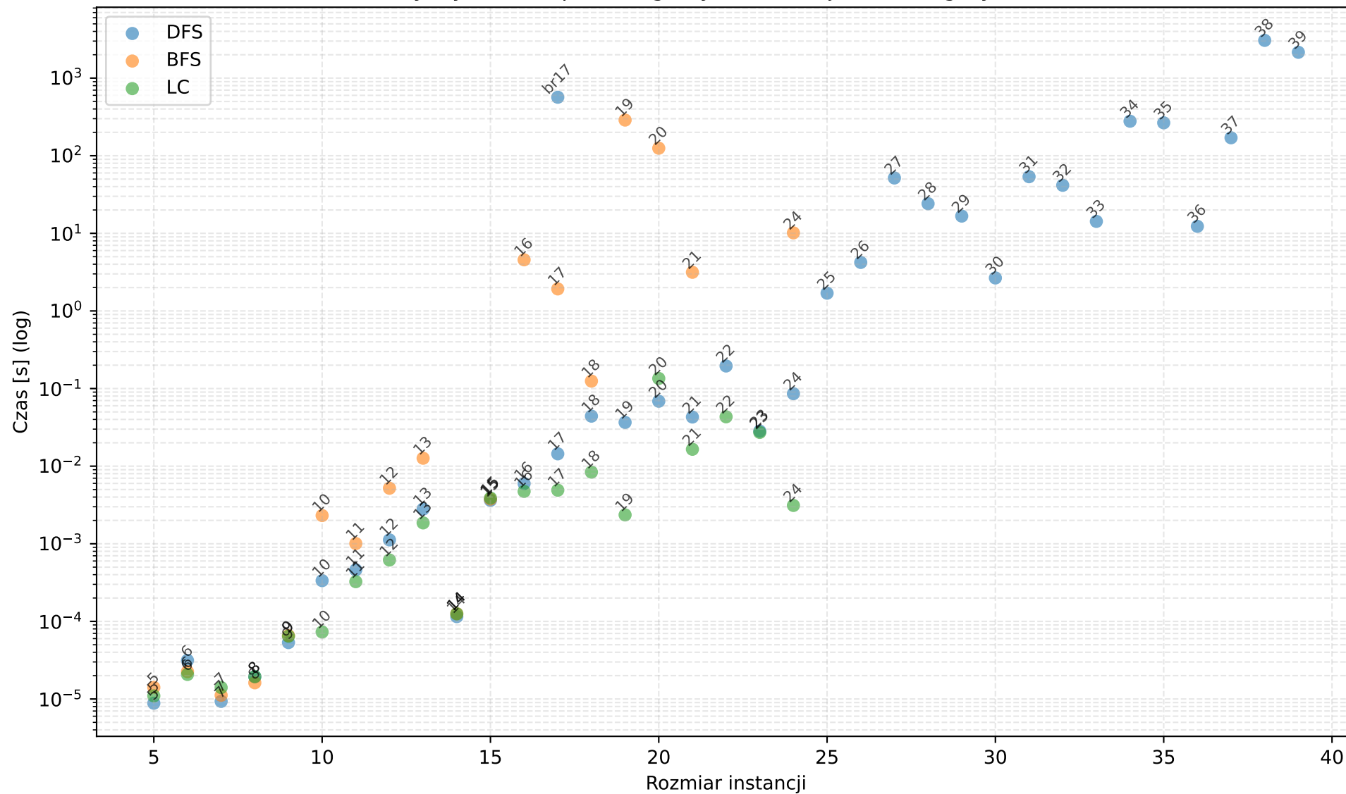
Czasy wykonania poszczególnych instancji (skala logarytmiczna)
