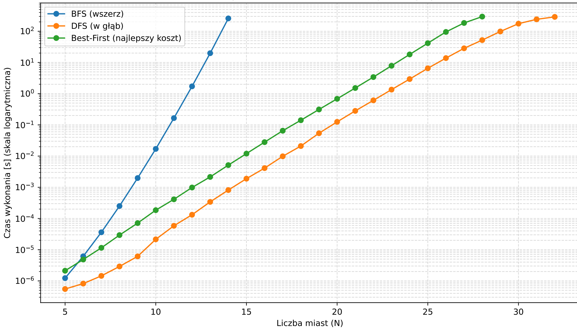
Zależność czasu wykonania od rozmiaru instancji dla algorytmu B&B
