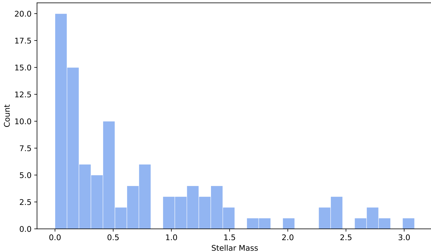
Stellar Mass PDF
