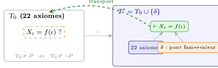
Figure 3: Le coup que seul un substrat où la théorie est une donnée permet. Lecture : chaque grand rectangle arrondi est une théorie (à gauche la référence T_0 , à droite son extension T' ) ; à l'intérieur, les boîtes bleues sont des axiomes, la boîte orange la définition \delta ajoutée (et, à gauche, l'hypothèse orange à laquelle elle répond), la boîte verte le but désormais démontrable ; la flèche verte en tirets est le transport du résultat en retour dans le langage de T_0 . Quand une hypothèse est indépendante (ici le pont famille-valeur, indépendant de A_{T_0} ), aucune recherche ne la ferme — le seul coup légal étend la théorie par une définition \delta , démontre l'image, et transporte le résultat en retour.
