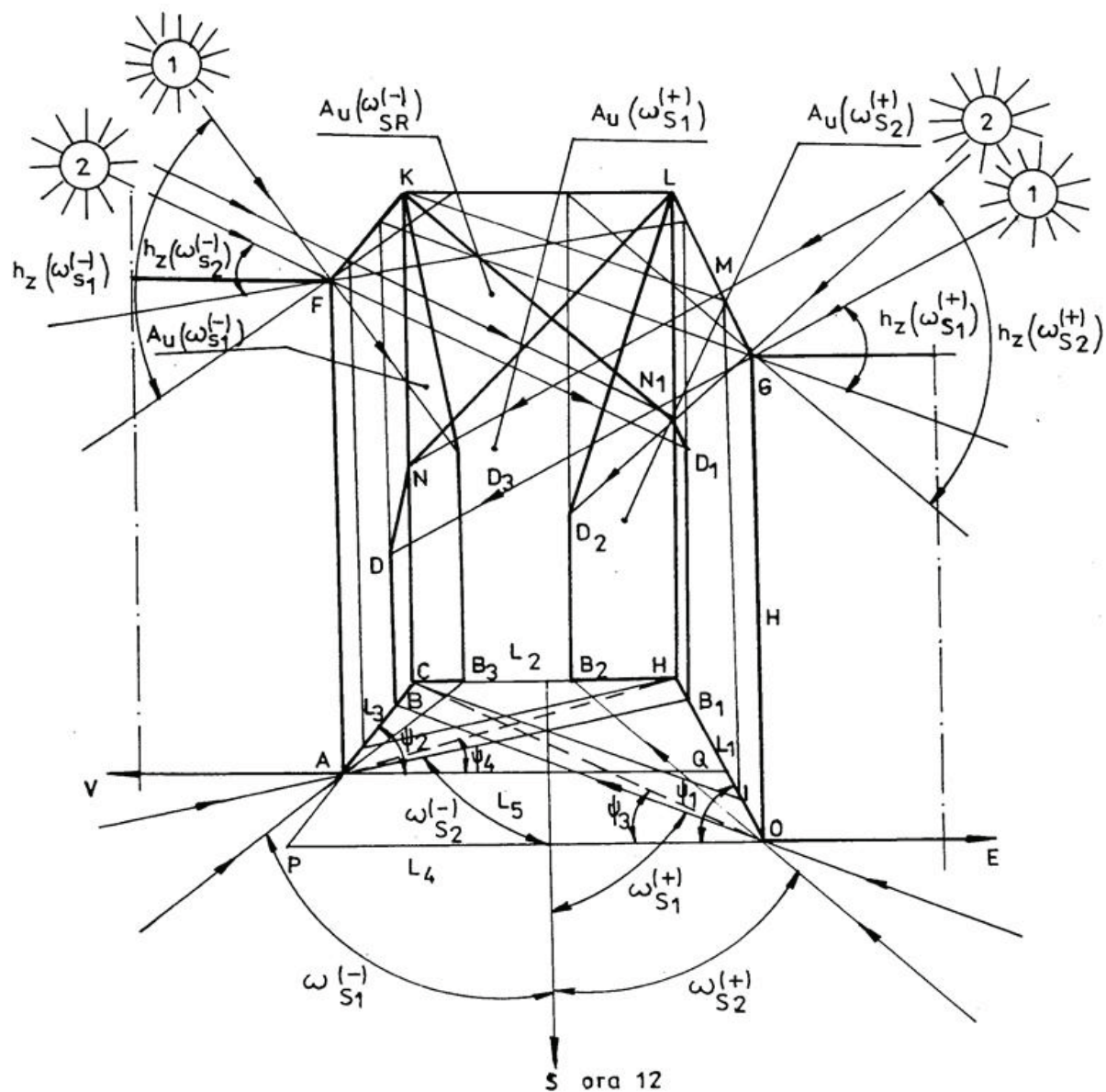
Fig. VI.3 – Schema de calcul al suprafeței afectate de umbră
