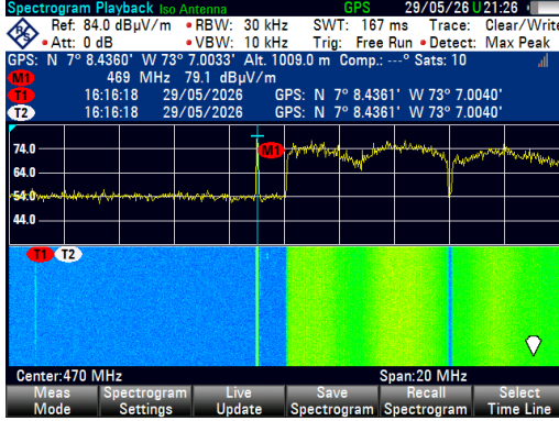
(a) Señal sin modulación.
