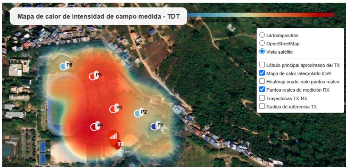
Figura 2: Mapa de calor construido a partir de las mediciones físicas.
