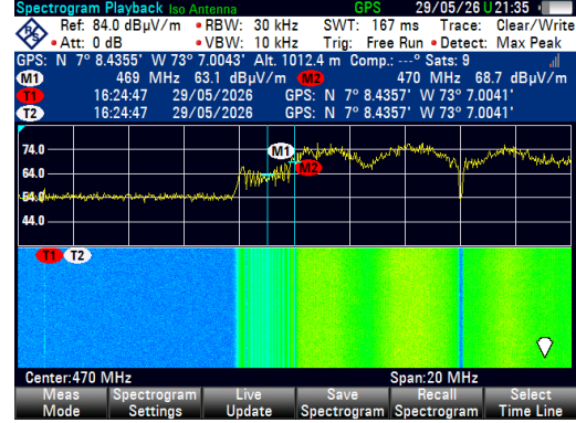
(b) Señal con modulación.
