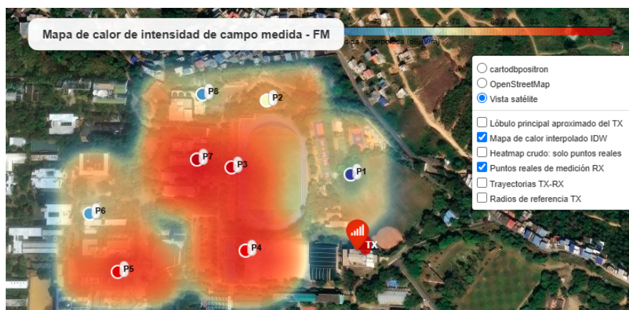
Figura 2: Mapa de calor construido a partir de las mediciones físicas en la banda FM.
