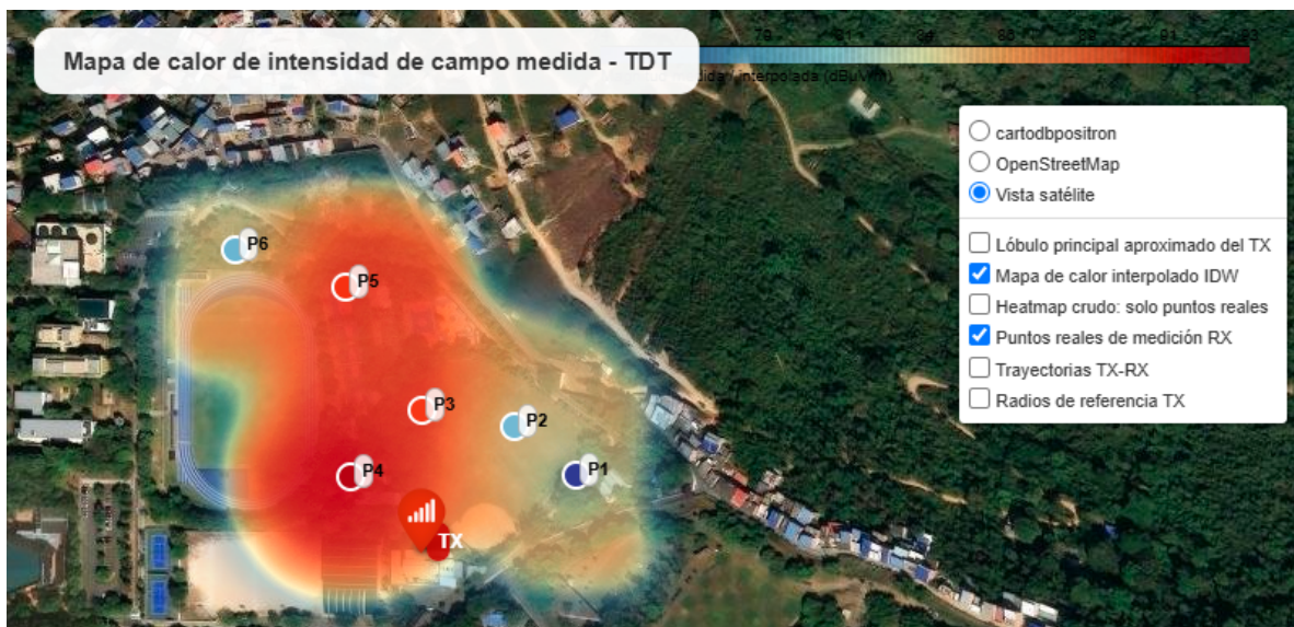
Figura 2: Mapa de calor construido a partir de las mediciones físicas.
