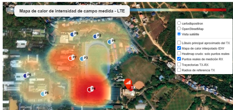
Figura 2: Mapa de calor construido a partir de las mediciones físicas en la banda LTE.
