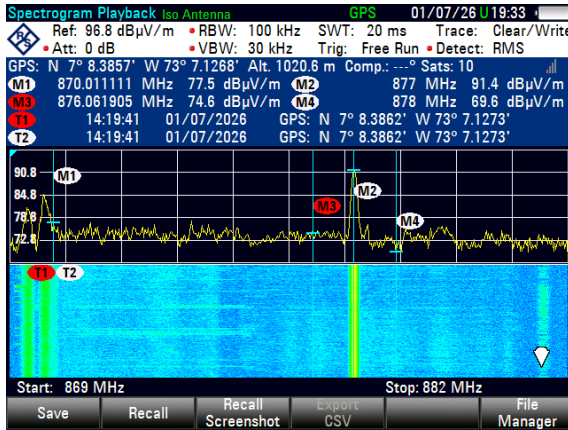
Figura 6: Comparación espectral de la señal interferente LTE en el punto de medición P4.
