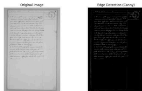
Fig.6 Edge Detection(Canny)
