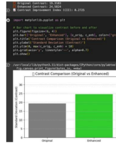
Fig.11 CII Result
