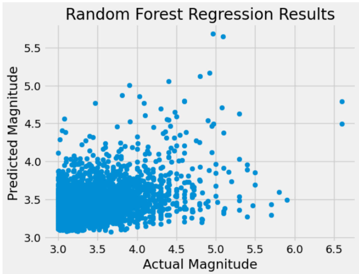
Actual vs Predicted
