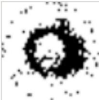
Loc
